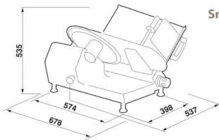
Rozměry GRAVINOX 350
