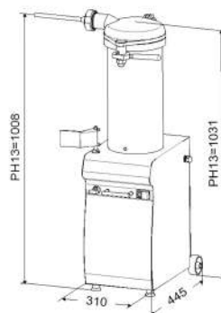
Rozměry PH13
