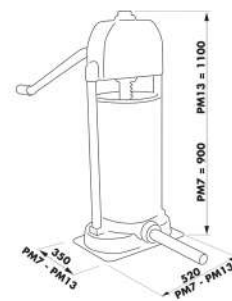
Rozměry PM7 & PM13
