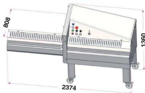
Rozměry ICÔNE 1100
