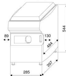
Rozměry Dimensions
