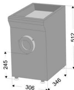
Rozměry 82 Classic Dimensions 82 Classic
