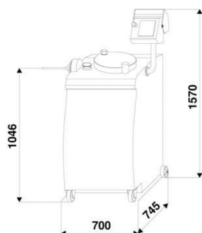
Rozměry TORSADO
